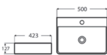
LOTUS PULTRA ÉPÍTHETŐ PORCELÁN MOSDÓ
