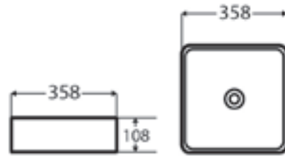
TULIP PULTRA ÉPÍTHETŐ PORCELÁN MOSDÓ
